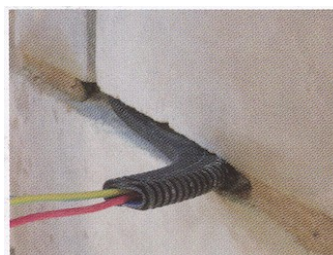
Exemple d'encastrement de conduit électrique dans des joints de pierre assisés
