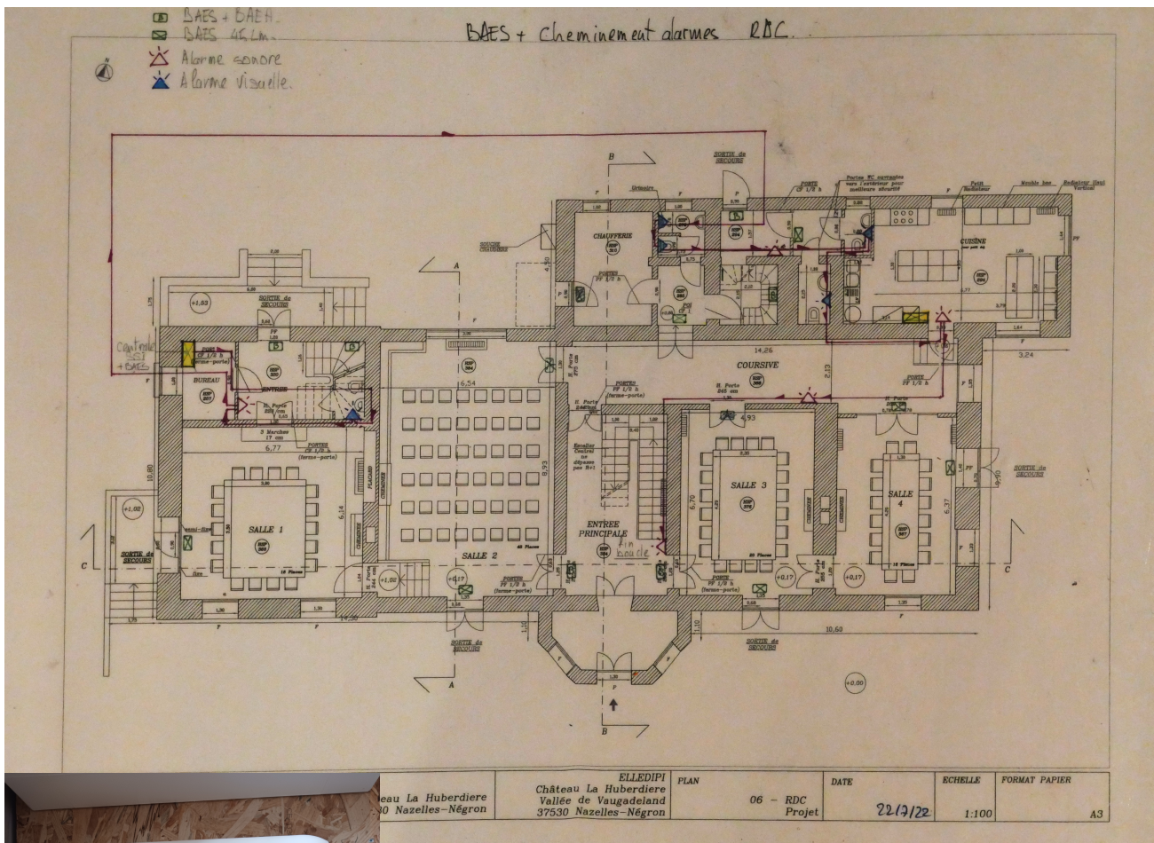
Exemple de plan SSI du rez de chaussée du château
